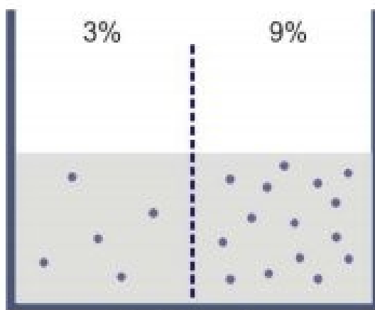
Semi-Permeabel membraan
